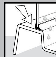
Allineare la parete al bordo interno del piatto doccia / Align the wall to the inner edge of the shower plate
