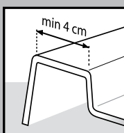
Larghezza del bordo piatto doccia \geq 4 cm Width of the border of the shower plate \geq 4 cm
